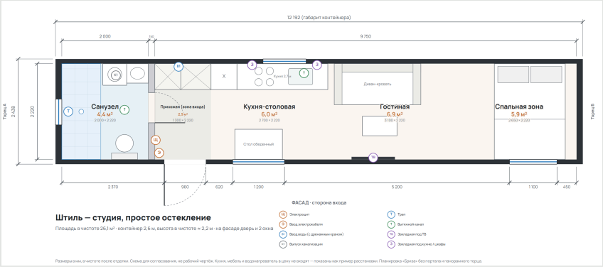
«Штиль» — студия, контейнер 2,6 м. Схема с мебелью — мебель и кухня в базовую цену не входят.
